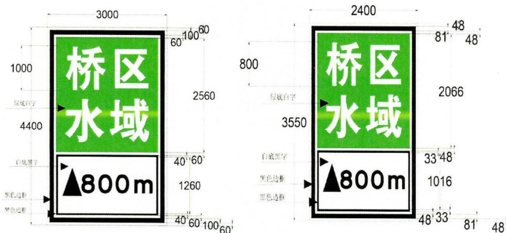
A 型（适合 IV 级及以上航道），尺寸单位：mm B 型（适合 V 级及以上航道），尺寸单位：mm
